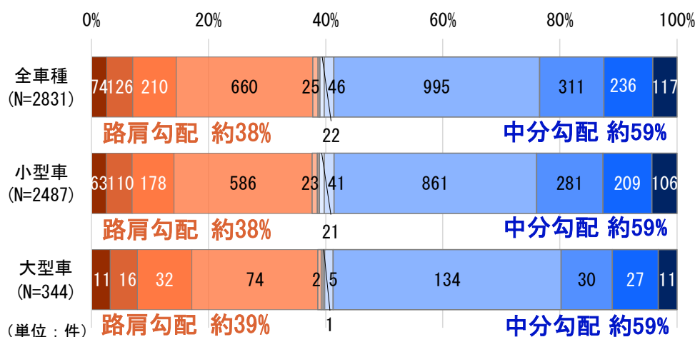
＜横断勾配別の接触事案発生件数＞
