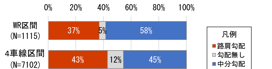
＜令和4年度 4車線区間との事故発生状況の比較＞
