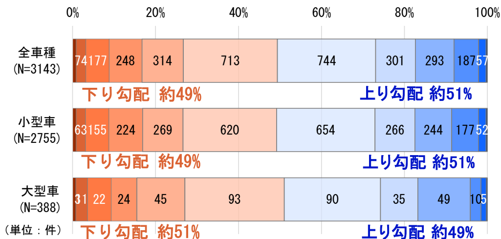
＜縦断勾配別の接触事案発生件数＞
